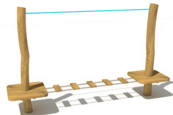
1 / BALANČNÍ SESTAVA - MŮSTEK
